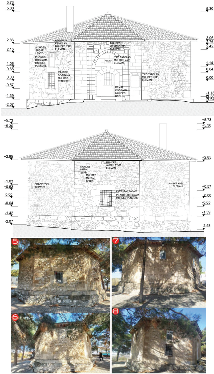
Şekil 12: Türbenin doğu ve batı cephelerinin rölövesi ve görselleri
