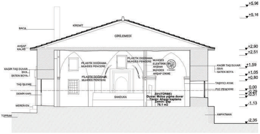
Şekil 7: İç mekânda giriş, sanduka, mihrap, ahşap dikme ve kalem işlerinin yerleşimi
