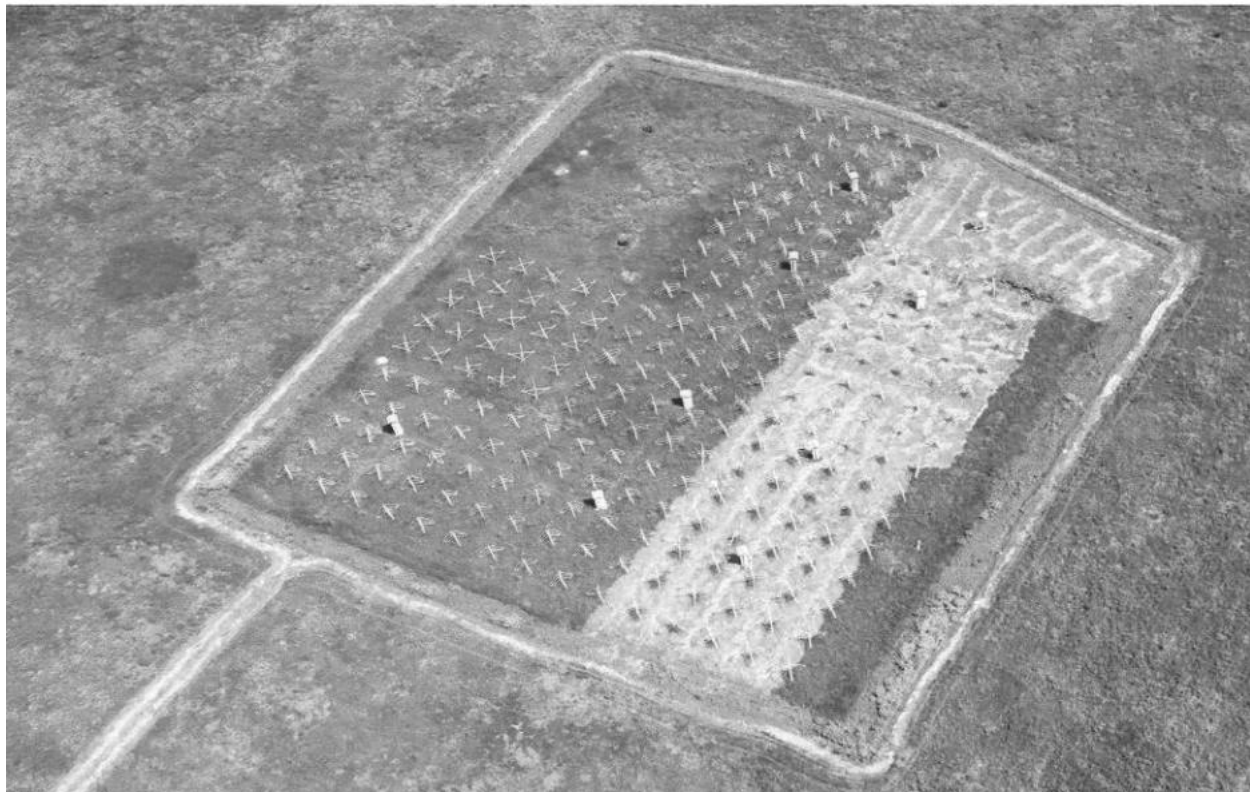
Рис. 23. Радіотелескоп нового покоління ГУРТ (9×25 двополяризованих елементів): зверху – зовнішній вигляд решіток, знизу – вигляд з квадрокоптера
