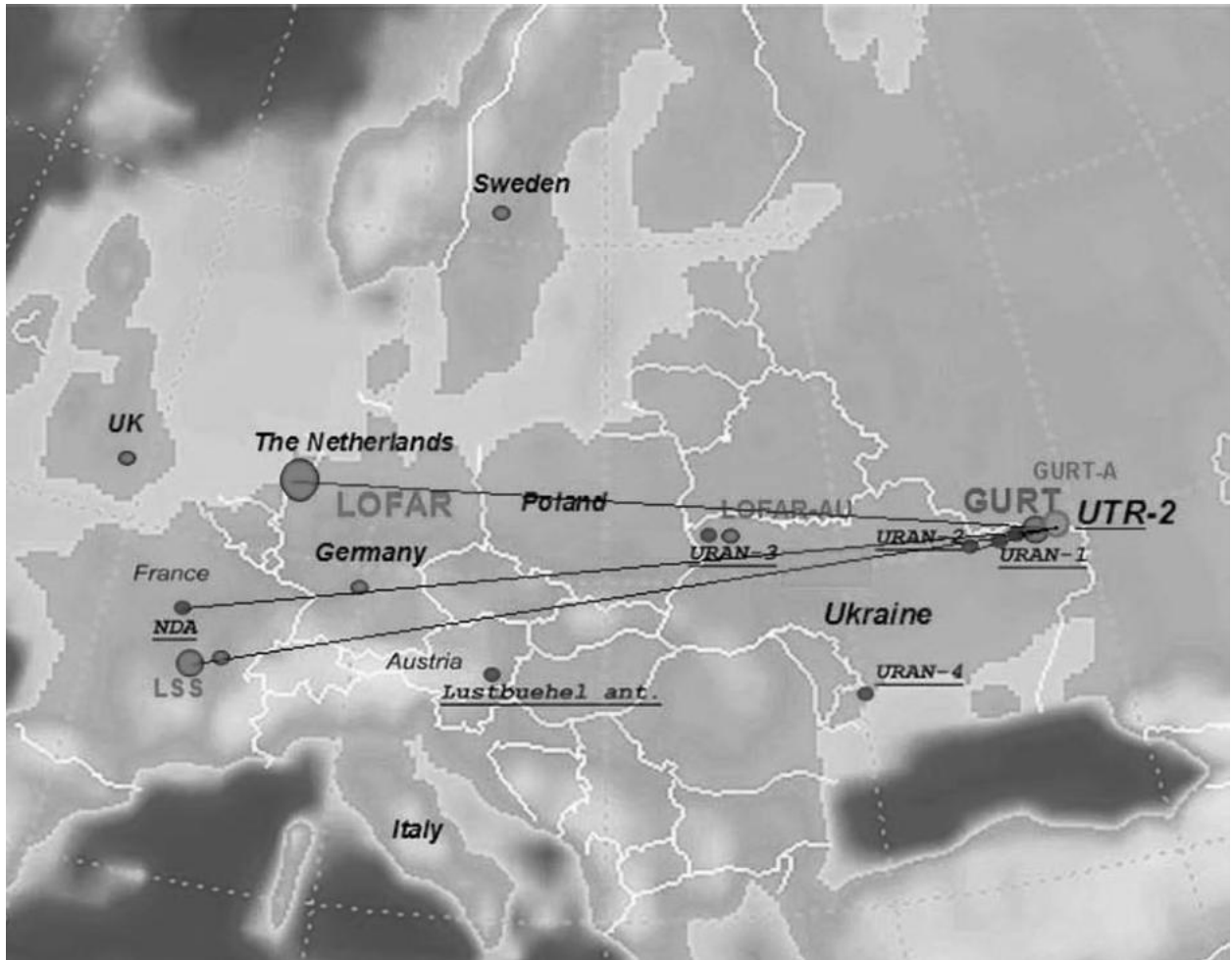
Рис. 48. Розташування сучасних низькочастотних радіотелескопів у Європі [32]
