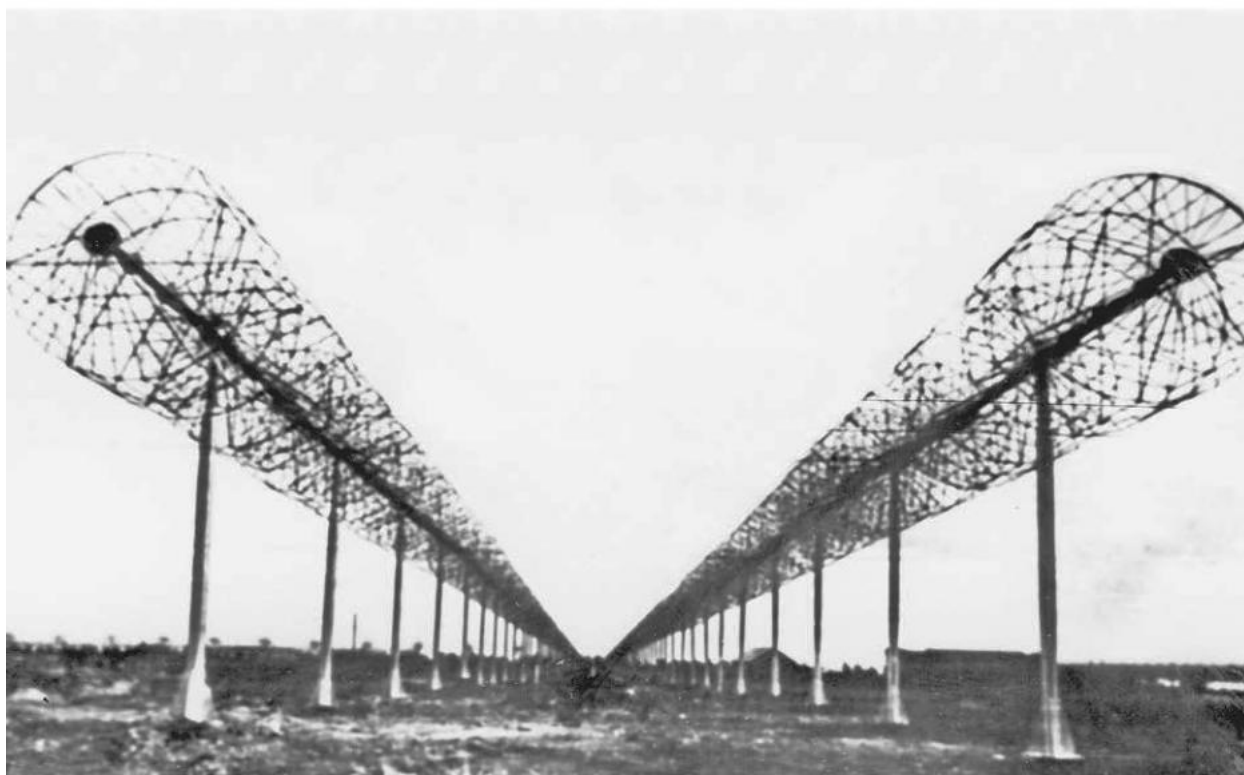
Рис. 4. Антени Північ–Південь і Схід–Захід радіотелескопа УТР-1 діапазону 10 \div 25 МГц – першого Т-подібного радіотелескопа у Європі
