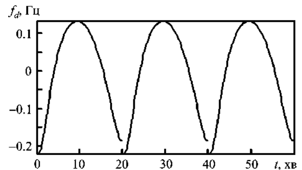
Рис. 9. Доплерограма вертикального зондування в с. Гайдари ( O -хвиля, |\Delta N|/N = 10\% , \psi = 90^\circ )
