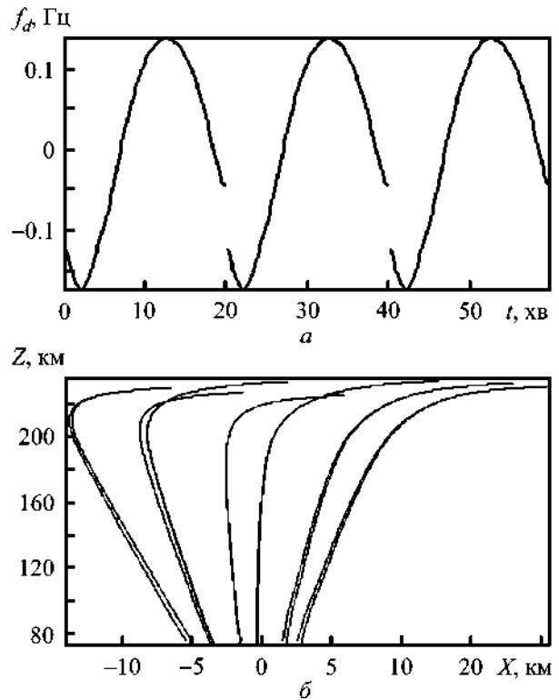
Рис. 8. Доплерограма (а) та проєкції траєкторій на вертикальну площину для O -хвилі (б) (РІЗ рухається похило уздовж геомагнітного меридіану, \delta = 10\% , довжина хвилі – 100 км, період – 20 хв)
