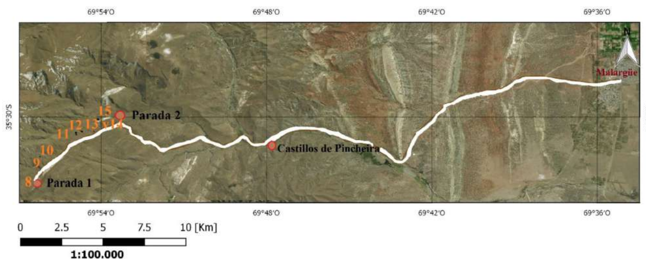
Figura 4. Georruta N.º 2 en camino a Castillos de Pincheira en zona sur, con paradas (geositios) y dolinas enumeradas de 8 a 15.
