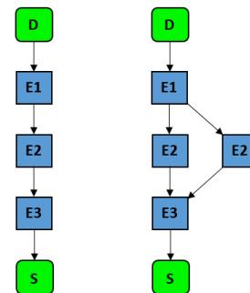
Fig. 6. Segmentación de Cauce con estados en serie y en paralelo.
