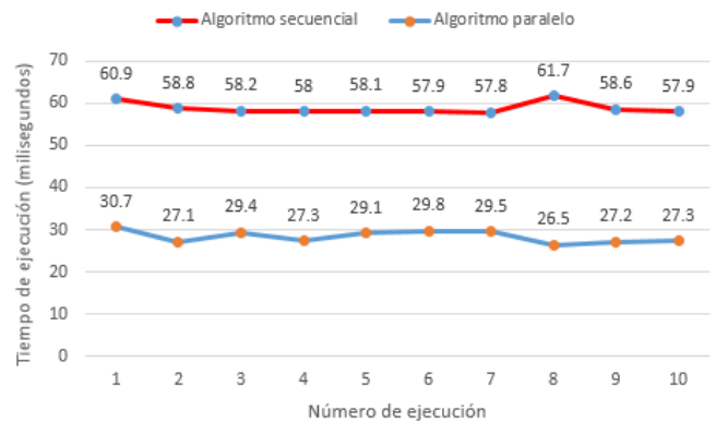
Fig. 9. Tiempo de ejecución del algoritmo secuencial y paralelo.
