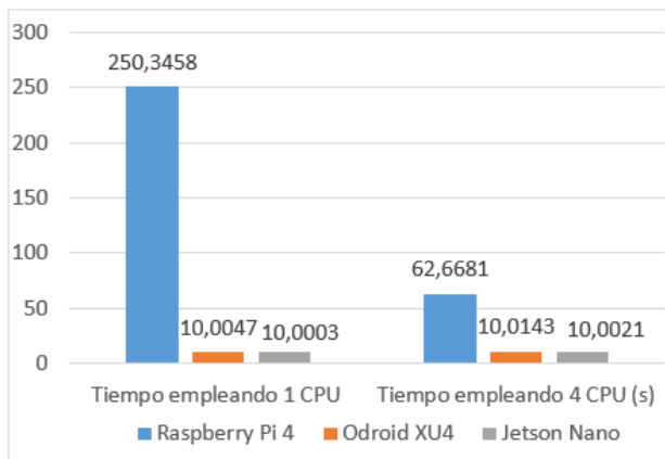
Fig. 3. Resultados de las pruebas de rendimiento a las unidades centrales de procesamiento.
