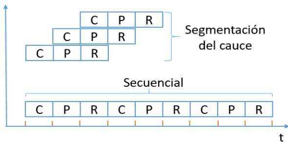
Fig. 7. Comportamiento en el tiempo del patrón segmentación de cauce.
