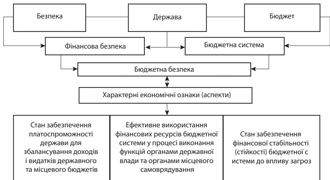
Рис. 1. Графічне подання терміна «бюджетна безпека»
