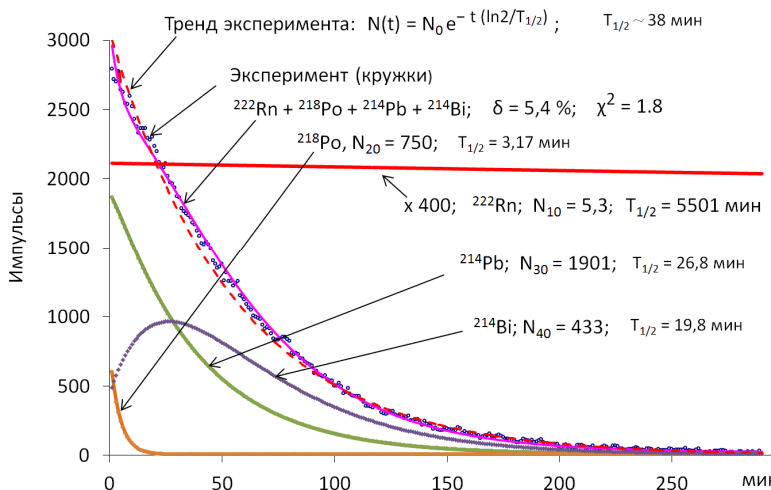
Рис. 1. Результаты измерения фильтра радиометром и обработка.
