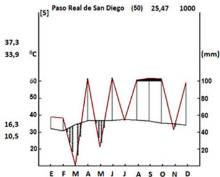
Figura 1. Diagrama climático del área en estudio.
