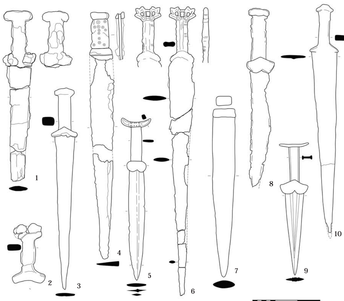
Рис. 13. Акинаки Нижнеднепровской группы: 1 - Арциз, к. 1, п. 13; 2 - Талмаза, к. 9, п. 1; 3 - Николаевка II, п. 8; 4 - Николаевка I, п. 3; 5 - Тудора-Паланка, п.; 6 - Пуркарь, к. 7, п. 3; 7 - Дивизия, к. 20, п. 6; 8 - Маяки, п. Г2; 9 - Дачное (Гниляково); 10 - Николаевка II, п. 7.
