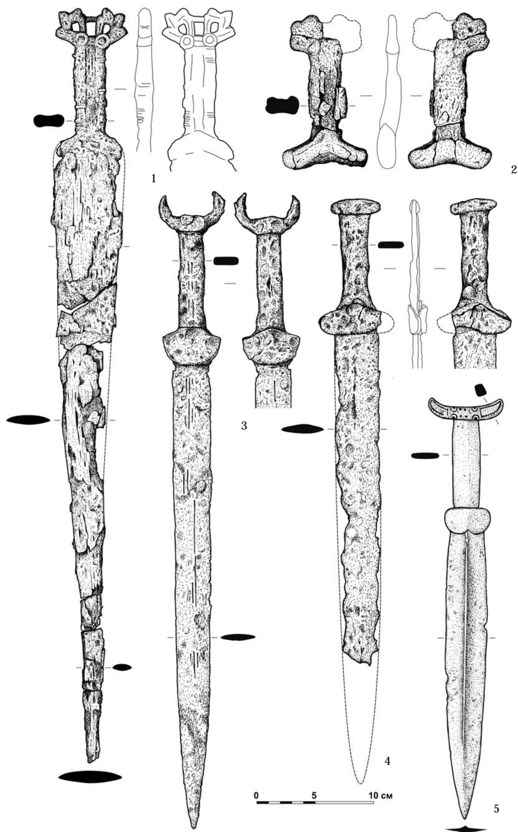
Рис. 1. Скифские мечи и кинжалы из комплексов Днестровско-Прутского междуречья (коллекция НМИМ): 1 - Пуркарь, к. 7, п. 3; 2 - Талмаза, к. 9, п. 1; 3 - Пыржолтень; 4 - Суручень; 5 - Олонештский район (Тудора-Паланка).
