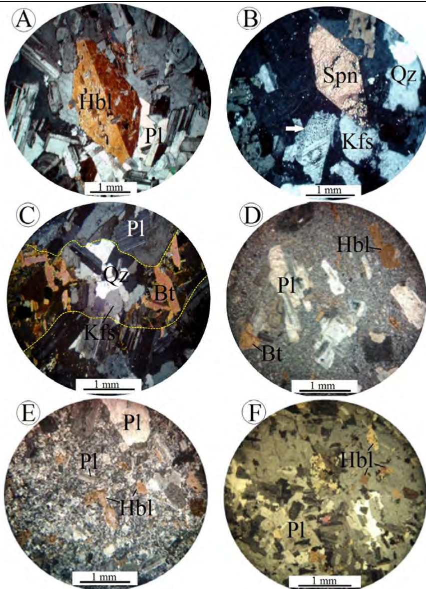
شکل ۳. تصاویر میکروسکوپی (نور عبوری پلاریزه متقاطع) از کانی‌های تشکیل‌دهنده و بافت واحدهای سنگی در منطقه قره‌چیلر، A: بافت‌های هتروگرانولار، مونزونیتی و پوئیکلیتیک همراه با بلور شکل‌دار هورنبلاند در توده گرانودیوریت-کوارتز مونزودیوریت، B: بافت میرمکتیکی (علامت فلش) همراه با بلور شکل‌دار اسفن در توده گرانودیوریت-کوارتز مونزودیوریت، C: بلورهای بیوتیت به همراه کوارتز و فلدسپار پتاسیم ثانویه در رگه‌چه‌های تیره‌رنگ که توده گرانودیوریت-کوارتز مونزودیوریت را قطع کرده‌اند، D: بافت پورفیری و فسوفیری در آپوفیز گرانیت پورفیری، E: بافت میکروگرانولار تا پورفیری در آپوفیز گرانیت پورفیری و F: بافت مونزونیتی و میکروگرانولار در استوک کوارتز مونزونیت. بلورهای شکل‌دار پلاژیوکلاز و هورنبلاند در تصویر مشخص است. علایم اختصاری کانی‌ها از ویتنی و اوانز (Whitney and Evans, 2010) اقتباس شده است. (Bt: بیوتیت، Hbl: هورنبلاند، Kfs: فلدسپار پتاسیم، Pl: پلاژیوکلاز، Qz: کوارتز، Spn: اسفن)
