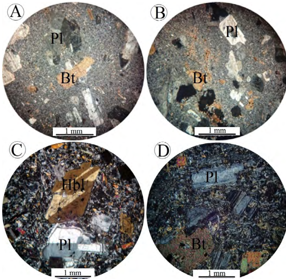
شکل ۵. A: بافت فسوفیری با درشت‌بلورهای پلاژیوکلاز حاوی منطقه‌بندی و بیوتیت در دایک‌های گرانیت پورفیری در منطقه قره‌چیلر، B: رگه‌چه‌های بیوتیت ثانویه موجود در دایک‌های گرانیت پورفیری، C: بافت پورفیری در دایک‌های آندزیتی حاوی درشت‌بلورهای پلاژیوکلاز و هورنبلاند و D: بافت میکروولیتیک پورفیری با درشت‌بلورهای پلاژیوکلاز و بیوتیت در دایک‌های تراکی‌آندزیتی. کلیه تصاویر در نور عبوری پلاریزه متقاطع گرفته شده‌اند. علائم اختصاری کانی‌ها از ویتنی و اوانز (Whitney and Evans, 2010) اقتباس شده است. (Bt: بیوتیت، Hbl: هورنبلاند، Pl: پلاژیوکلاز)
