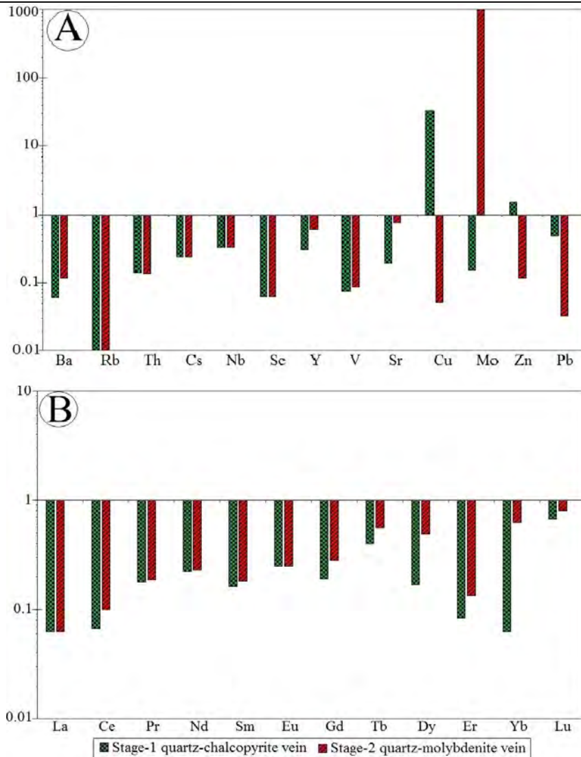
شکل ۱۳. A: نمودار عناصر کمیاب برای رگه‌های کوارتز کانه‌دار در رخداد معدنی قره‌چیلر که نسبت به توده گرانودیوریت- کوارتز مونزودیوریت دگرسان شده (نمونه QA-12، جدول ۱) بهنجار شده‌اند و B: نمودار عناصر کمیاب خاکی برای رگه‌های کوارتز کانه‌دار در رخداد معدنی قره‌چیلر که نسبت به توده گرانودیوریت- کوارتز مونزودیوریت دگرسان شده (نمونه QA-12، جدول ۱) بهنجار شده‌اند.
