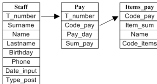
Рис.1. Спрощена структура БД «Заробітня палата»
