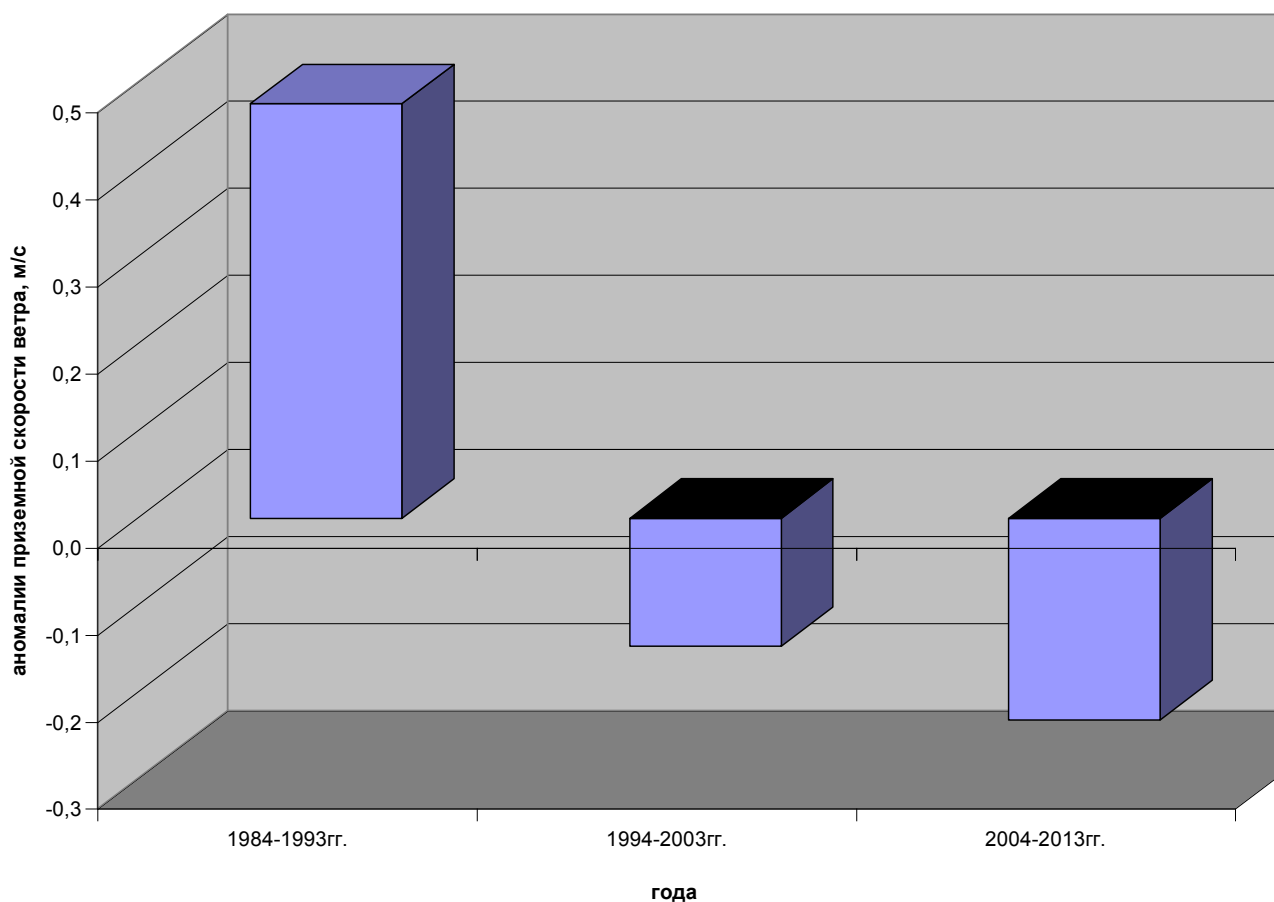
Рисунок 5. Суммы аномалий приземной скорости ветра по десятилетиям.
