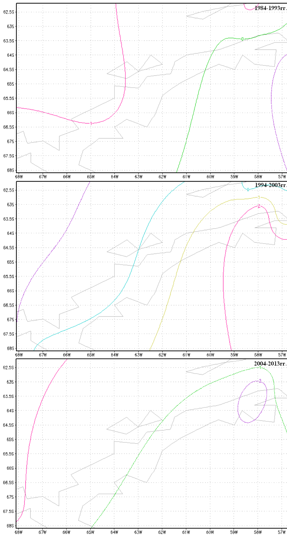
Рисунок 2. Пространственно–временное распределение аномалий приземной скорости ветра (апрель).
