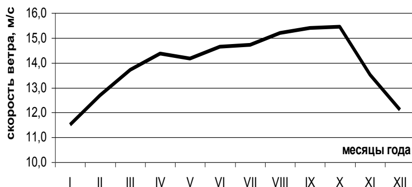
Рисунок 2. Годовой ход осредненных по территории среднемесячных значений приземной скорости ветра.
