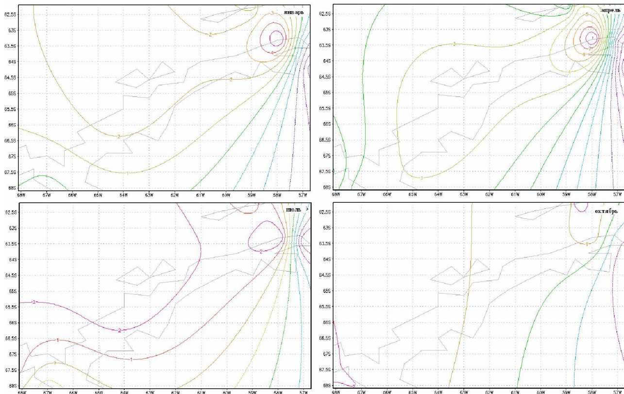
Рисунок 4. Картосхемы трендовой составляющей приземной скорости ветра для центральных месяцев сезонов.
