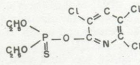
Chlorpyrifos
