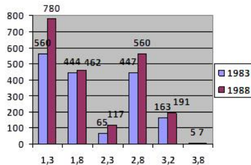
Рис. 10. Количество соударений (по вертикали) в диапазонах усилий (по горизонтали, МН)
