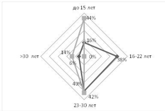
Рис. 2. Состояние парка окатышевозов по срокам эксплуатации
