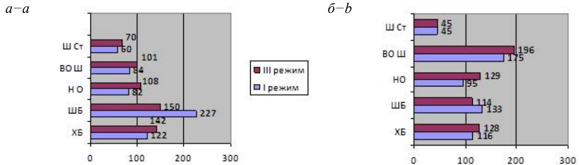
Рис. 8. Суммарные напряжения (по горизонтали, МПа) в элементах конструкции вагонов
