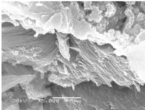
Рис. 9. Морфологія цементного каменю бездобавочного бетону на основі портландцементу марки ПЦ I 500Н (28 доба тужавіння), \times 5000
