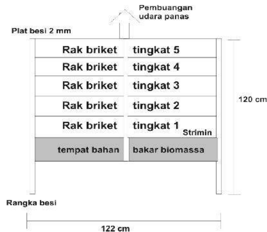
Gambar 1 Desain Alat Pengering- Tray Dryer Berbahan Bakar Biomassa
