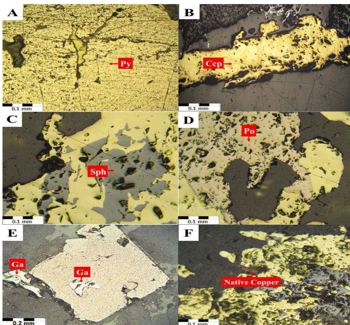
شکل 4. کانیهای فلزی بر اساس فراوانی در کانسار مس جیان: A: پیریت (Py)، B: کالکوپیریت (Ccp)، C: اسفالریت (Sph)، D: پیرویت (Po)، E: گالن (Ga)، F: مس خالص (Native Copper)
