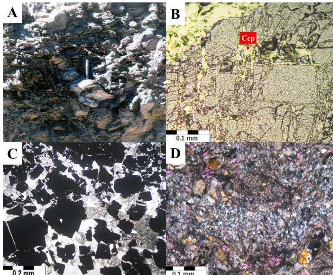
شکل 6. اثرات دگرگونی دینامیکی در کنسار مس جیان (A: بودیناژ در رگه‌های کوارتزی، B: پرشدگی رگه‌های پیریت به‌وسیله کالکوپیریت (Ccp)، C: بافت پرشی در نور عبوری، D: شیستوزیته و چین‌خوردگی در مقیاس میکروسکوپی).
