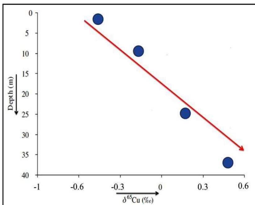
شکل 11. تغییرات \delta^{65}\text{Cu} کانیه‌های ثانویه مس نسبت به عمق در کانسار مس جیان.
