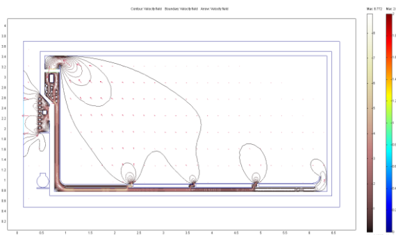
Рисунок 2 – Розрахункова модель холодильного рефрижераторного контейнера і поле швидкості повітря без завантаження
