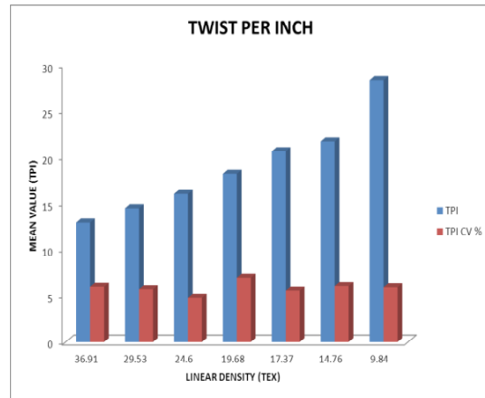
Fig. 1: TPI & CV%
