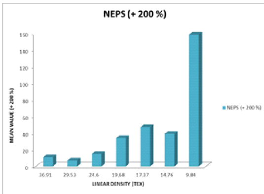
Fig. 11: Neps (+200 %)
