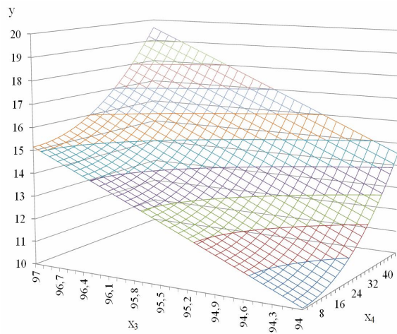
Рис. 3 - Зависимость сокращения времени легирования расплава с использованием металлизированного вторичного сырья, % (y) от степени усвоения молибдена и вольфрама при выплавке стали, % ( x_3 ) и содержания обожженного молибденового концентрата в шихте, % мас. ( x_4 )
