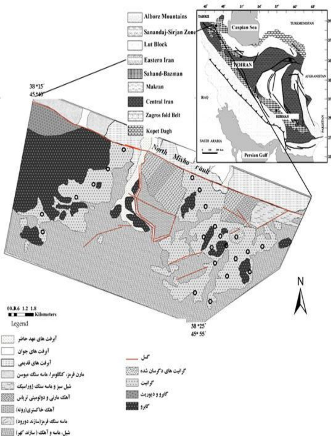
شکل 1. نقشه زمین‌شناسی منطقه مطالعاتی که بر پایه تصاویر ماهواره‌ای و نقشه 1/100000 مرنده تهیه شده است [5].
