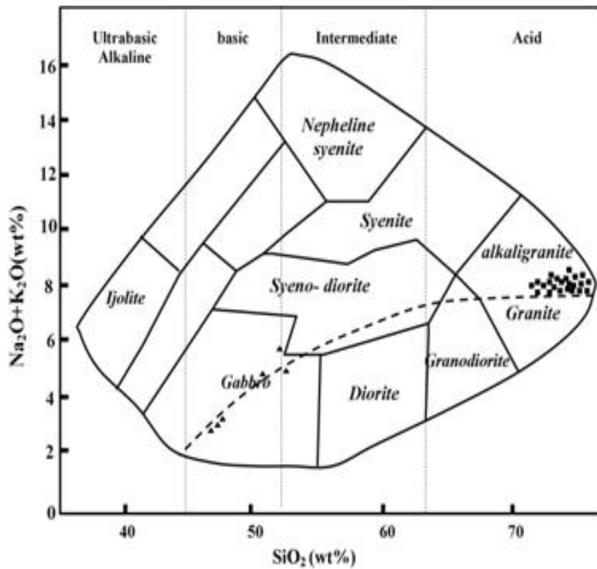
شکل 6. نمودار تغییرات \text{Na}_2\text{O}+\text{K}_2\text{O} در مقابل \text{SiO}_2 نمونه‌های فلسیک در محدوده آلکالی‌گرانیت و نمونه‌های مافیک در محدوده گابرو پلات می‌شوند [9 و 10]. مربع = فلسیک و مثلث = مافیک
