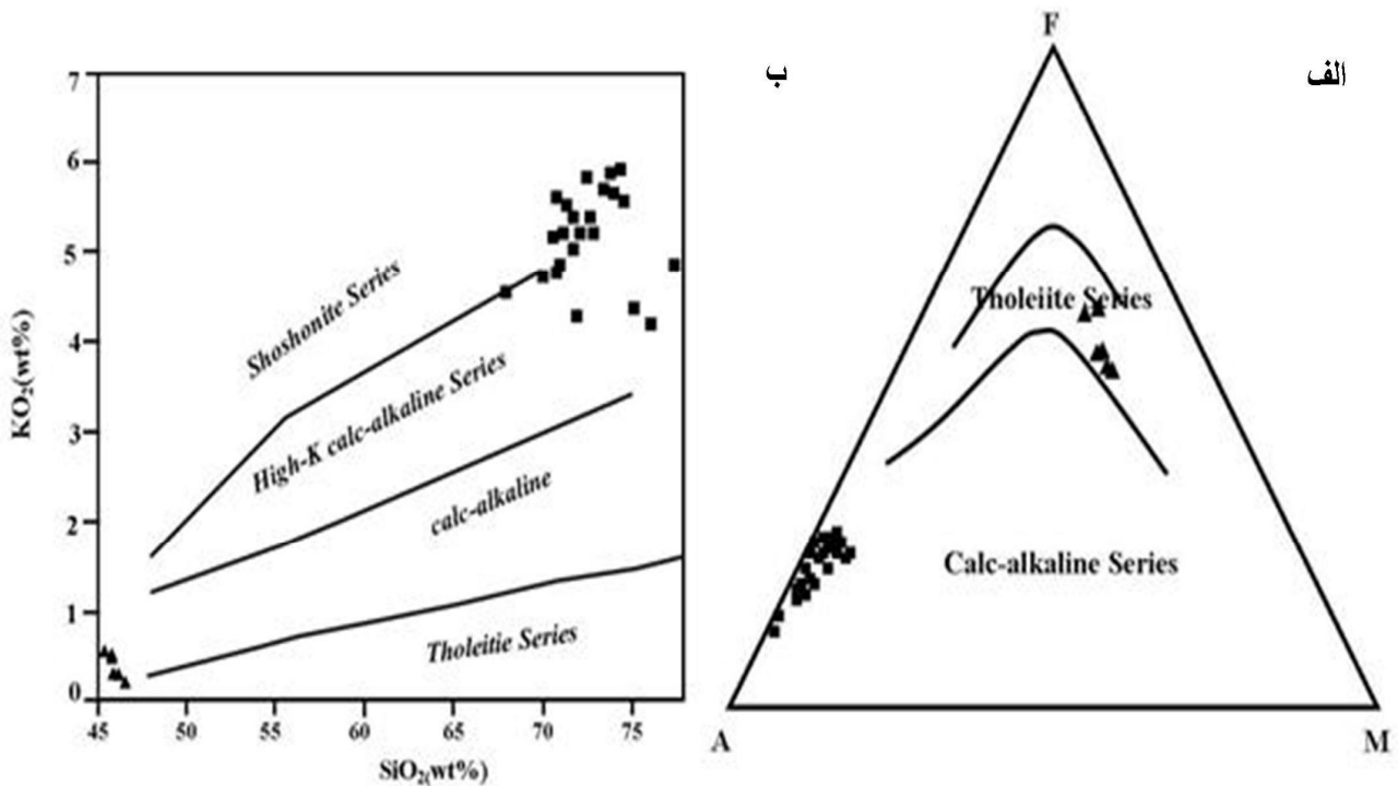
شکل 7. الف) نمونه‌های گرانیتوئیدی و بازیک در نمودار AFM [11]، ب) در نمودار \text{K}_2\text{O} در مقابل \text{SiO}_2 نمونه‌های اسیدی و گابرو به ترتیب در قلمرو کالکوالکالین غنی از پتاسیم و تولیتی قرار می‌گیرند [12].
