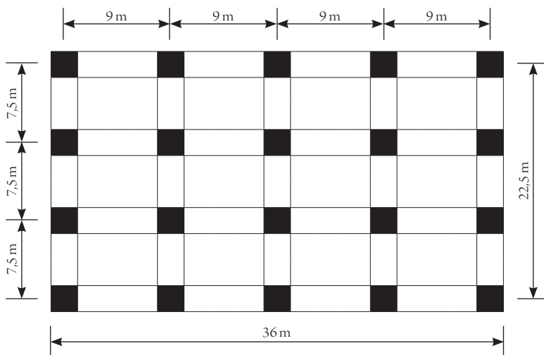
Figura 1. Planta típica
