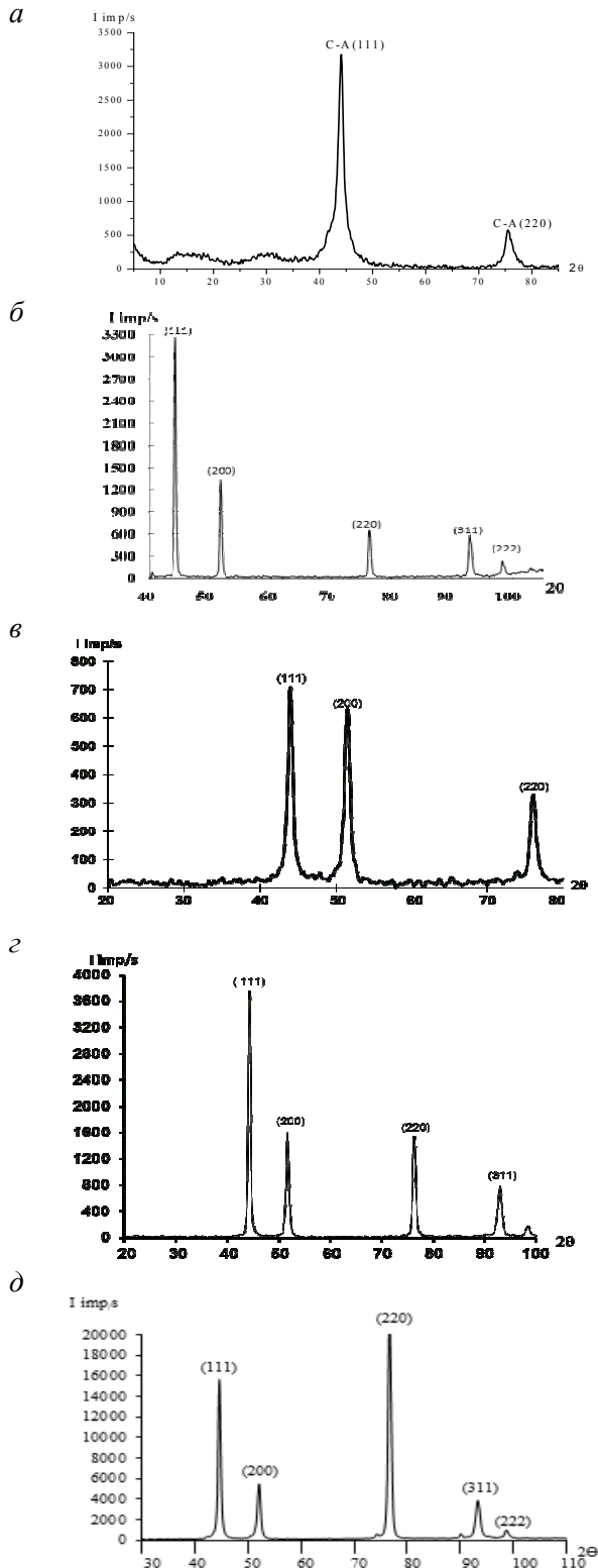
Рис. 4. Дифрактограми:
