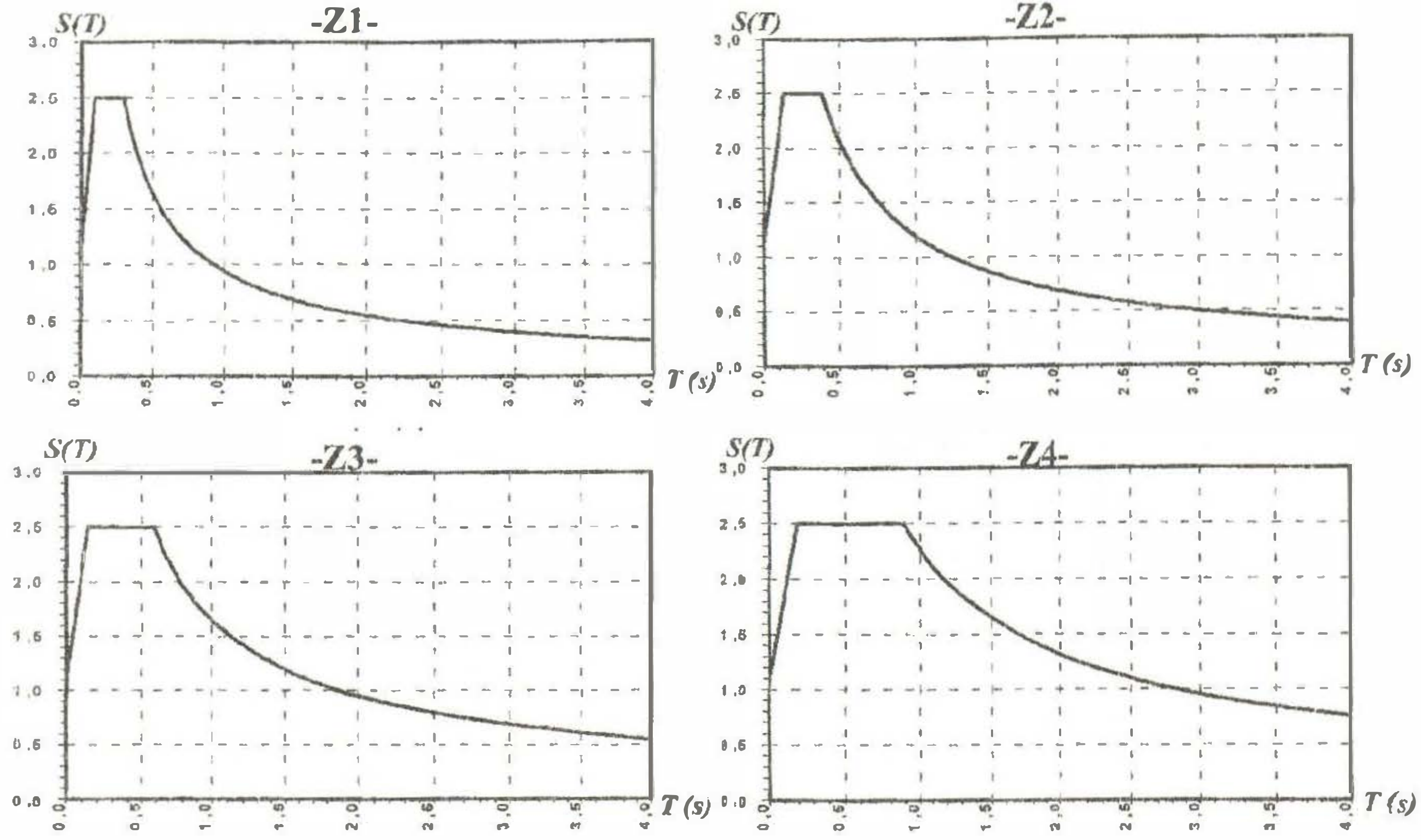
Şekil 3. Zemin sınıflarına göre spektrum katsayısının değişimi
