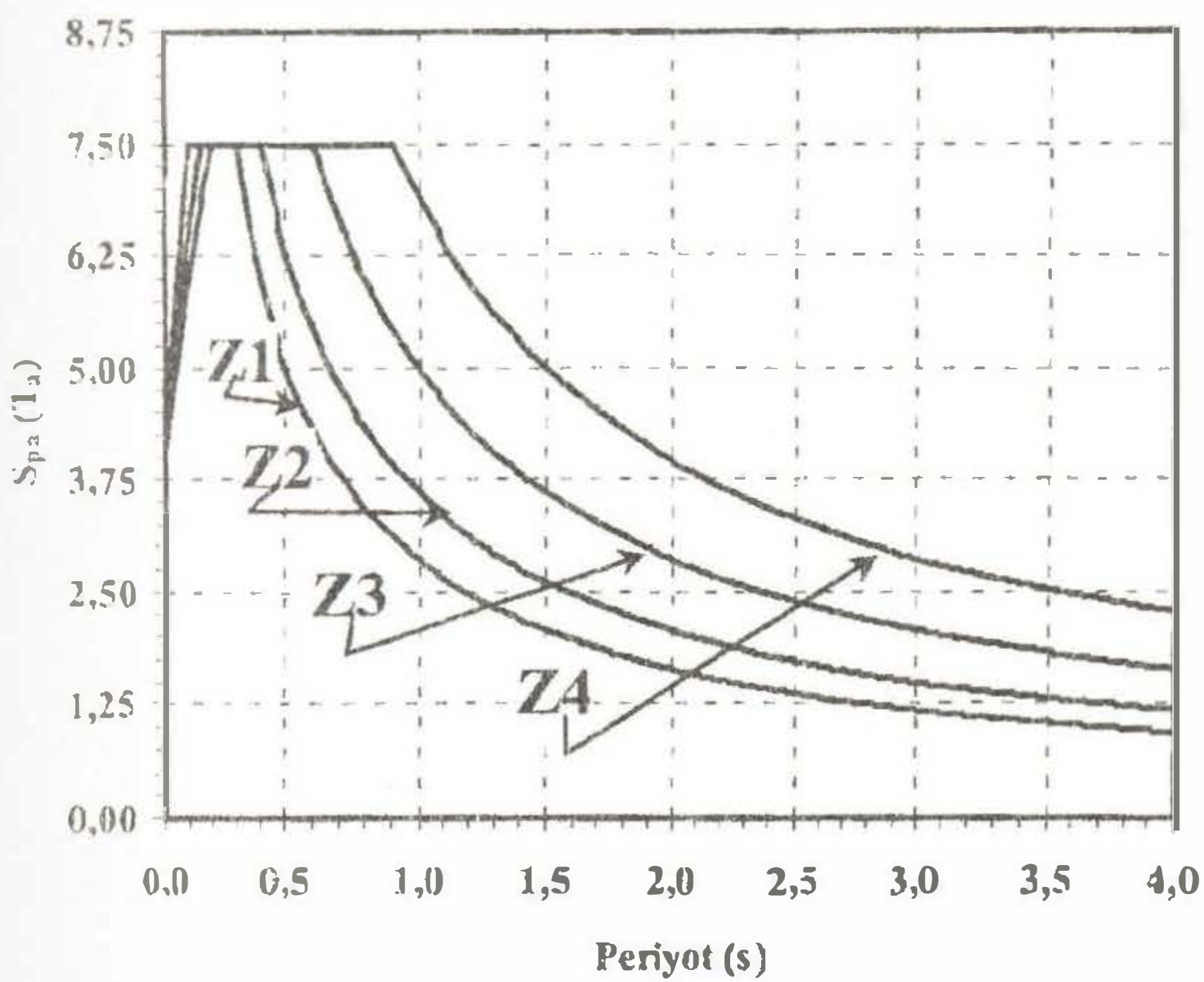
Şekil 4. Çalışmaya konu depolar için alınacak ivme spektrumları
