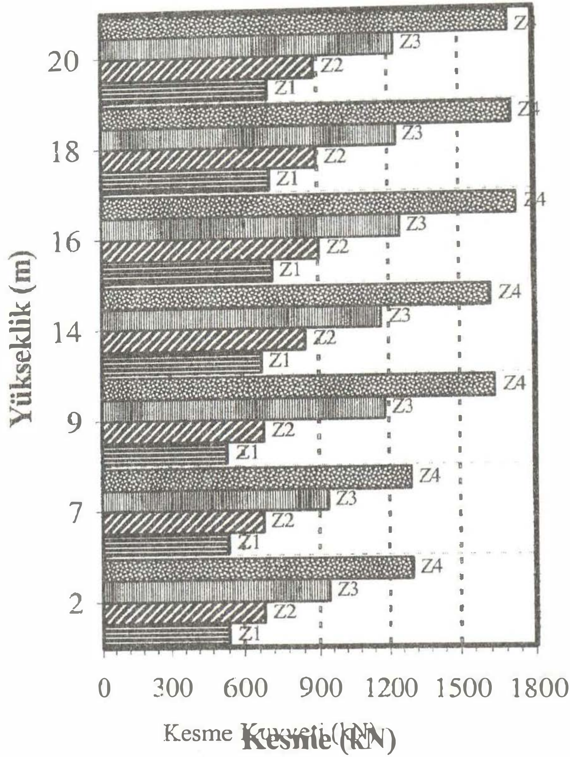
Şekil 10. Çerçeve sistemli deponun dikey taşıyıcı elemanlarındaki, farklı zemin koşulları için maksimum kesme kuvveti değişimi.
