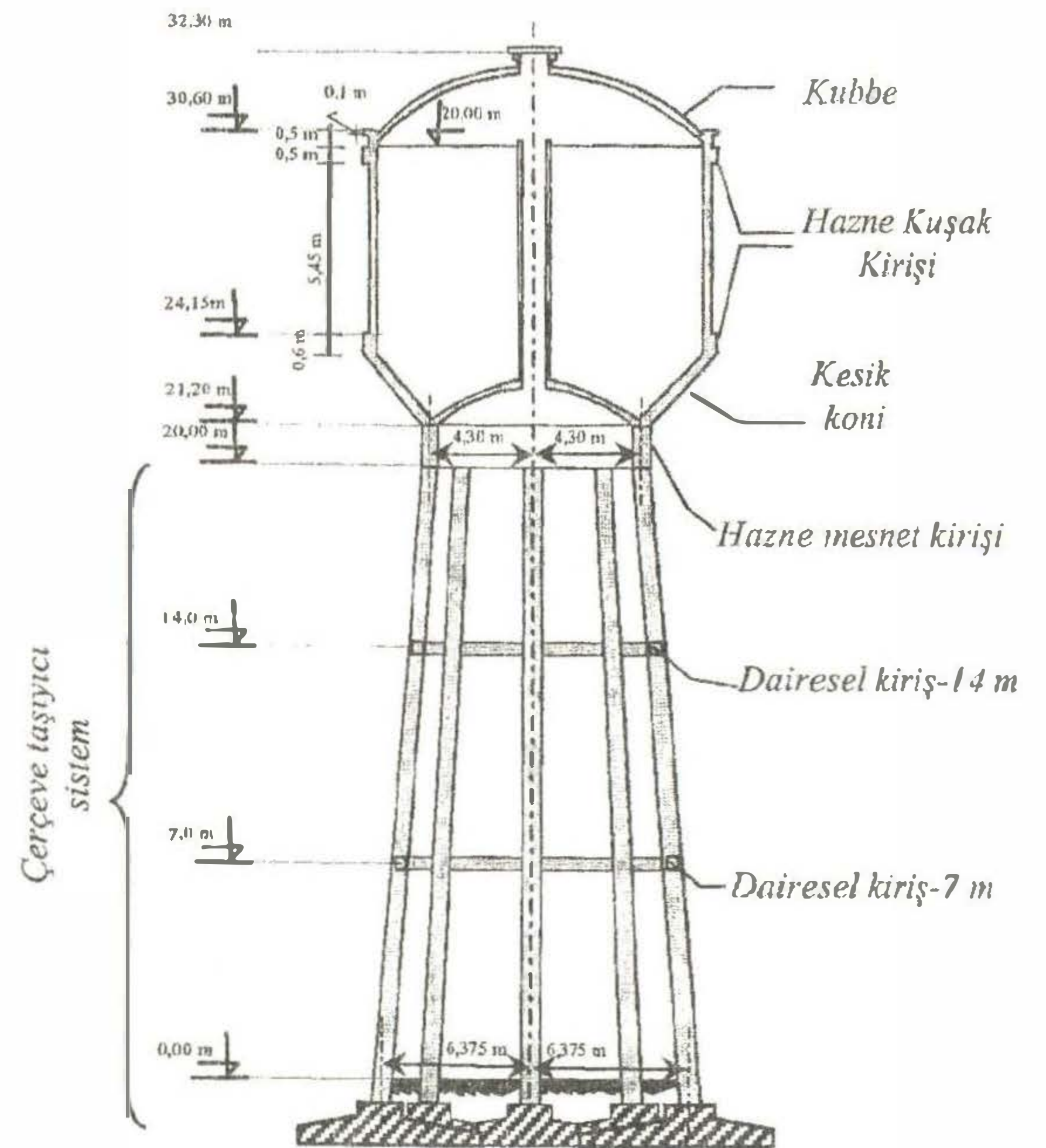
Şekil 5. Çerçeve taşıyıcı sisteme sahip deponun düşey kesiti
