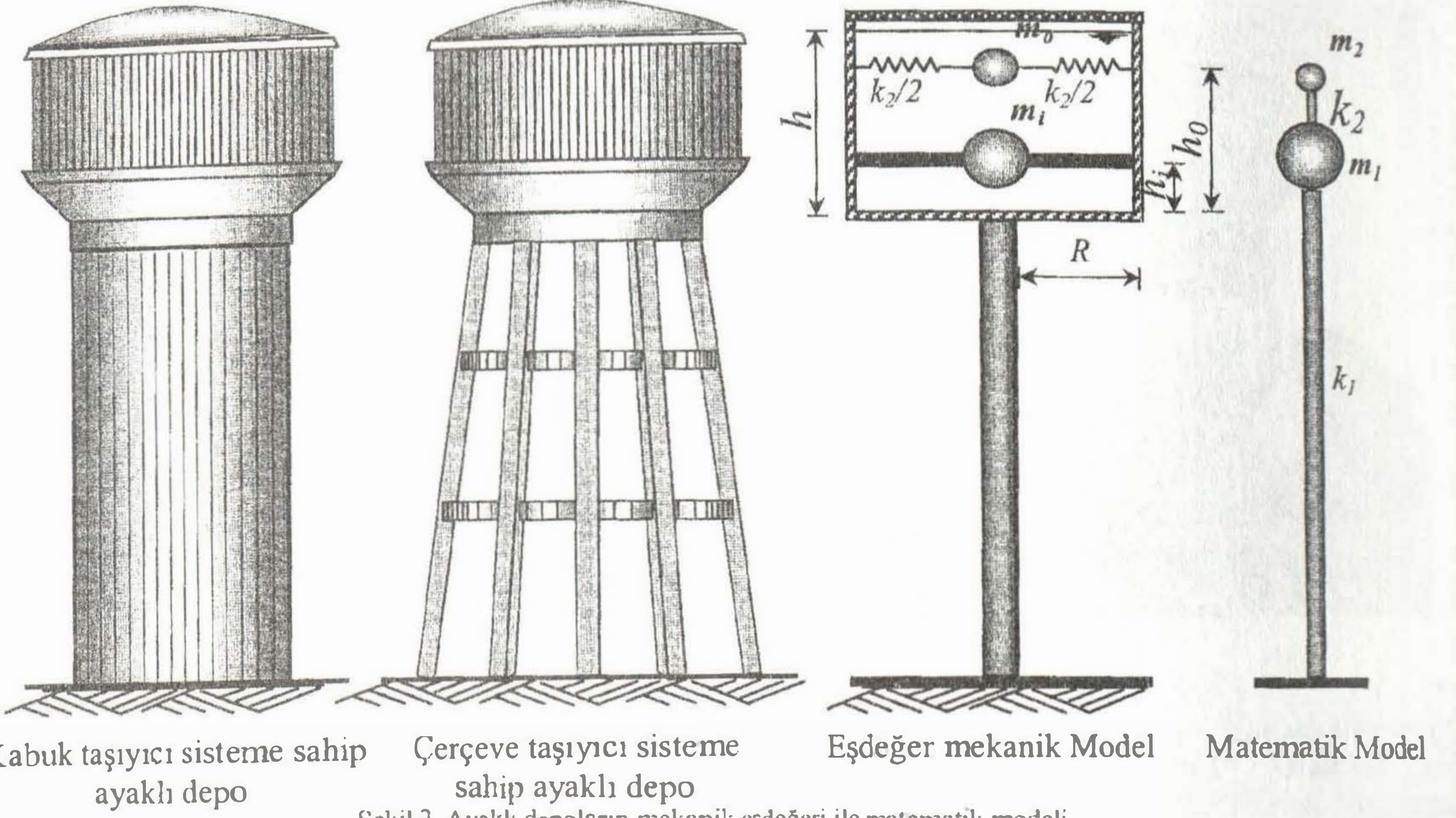
Şekil 2. Ayaklı depoların mekanik eşdeğeri ile matematik modeli
