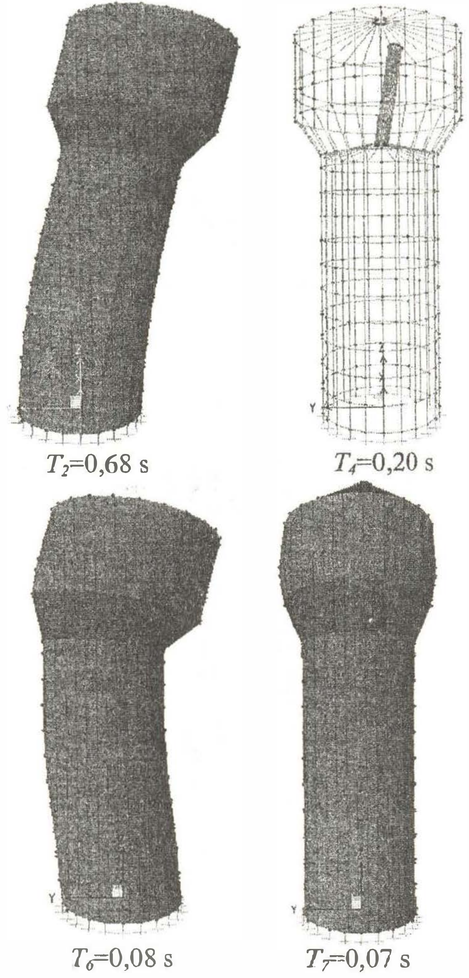
Şekil 8. Silindirik kabuk sistemli ayaklı deponun 4 farklı mod şekli ve periyotları
