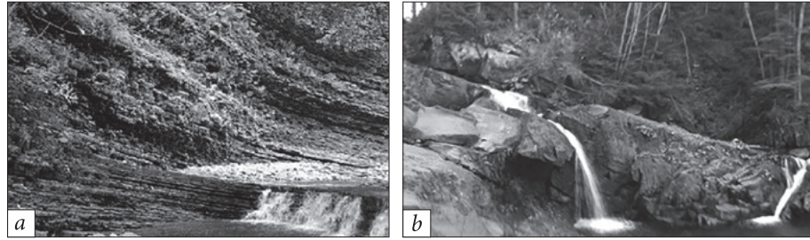
Рис. 1. Відслонення флішу Чорногірського (а) та кристалічних порід Мармароського масивів (b) Fig. 1. Outcrop of flysch of the Chornohirsky (a) and crystalline rocks of the Marmarosky massifs (b)
