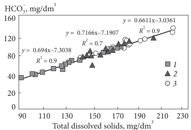
Рис. 5. Графік залежності між мінералізацією та HCO 3 - у водах річок: 1 — Лужанка, 2 — Велика Уголька, 3 — Мала Уголька
