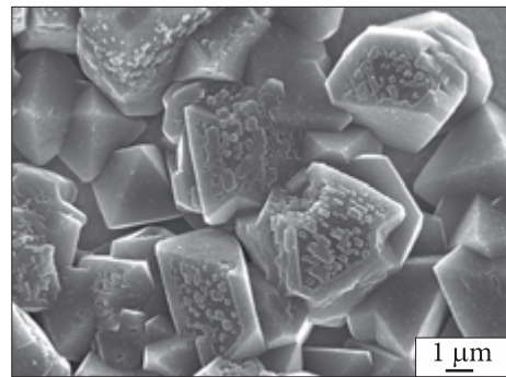
Рис. 4. Нарости нанометрових гладкогранних октаедрів і кубо-октаедрів діаманту на мікрметрових октаедрах CVD діаманту. Прояв автоепітаксії нанокристалів. ПЕМ знімок (JSM 6700F; SEI; 15,0 kV; WD 7,0 mm)
