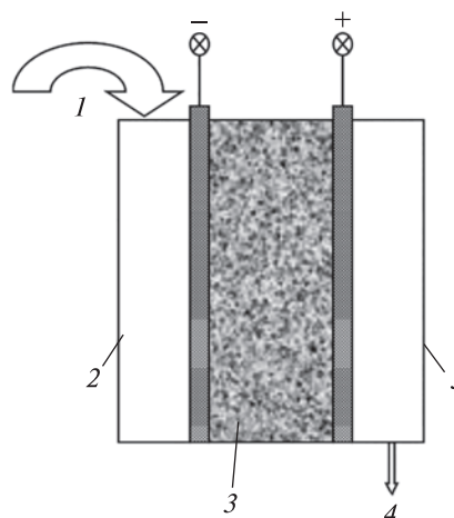
Рис. 1. Схема експериментальної електроосмотичної комірки: 1 – подача електроліту, 2 – анодна камера, 3 – роздільна мембрана, 4 – колектор фільтрату, 5 – катодна камера
