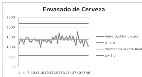
Figura 5. Validación del modelo de simulación con envasado de cerveza. Fuente: Elaboración Propia.
