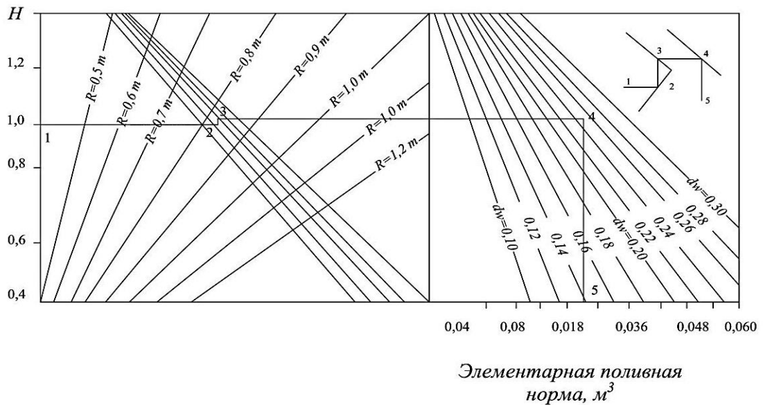
Рисунок 1. Номограмма для определения элементарной поливной нормы при очаговом увлажнении в системе капельного орошения.
