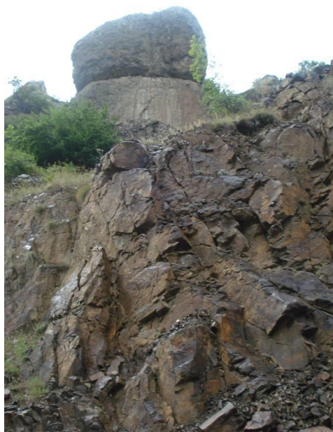
Рис. 3 Обвальний матеріал на склоне Муровдагського хребта
