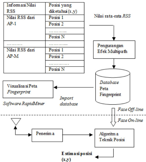
Gambar 3. Arsitektur sistem localization
