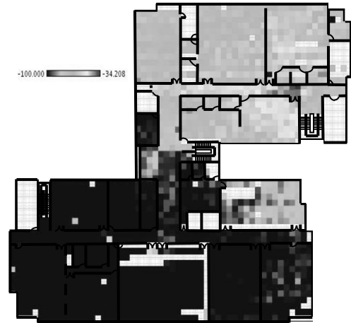
Gambar 8. Visualisasi peta fingerprint pada AP-4
