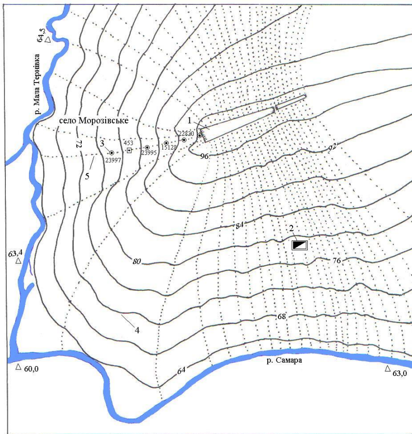
Рис. 1. Гідродинамічна сітка на ділянці «Балка Стуканова»
