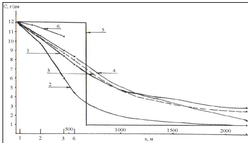
Рис. 3. Результати епігнозних розрахунків по створу ставок «Балка Стуканова» – ріка Мала Тернівка: 1 – режимні спостереження; 2 – D=3,0 м 2 /добу; 3 – D=25,0 м 2 /добу; 4 – D=30,0 м 2 /добу; 5 – «поршневе витіснення»; 6 – схема «Ловер'є» при D_m=5 \cdot 10^{-5} м 2 /добу
