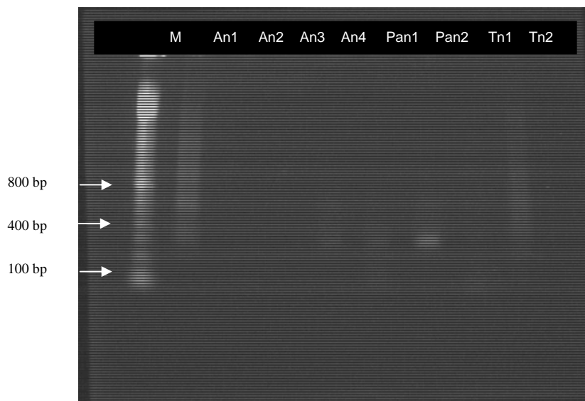
Gambar 4. Hasil amplifikasi PCR pada nyamuk Anopheles yang diduga filaria yang berasal dari bag. Parasitologi KUI dan pool nyamuk yang berasal dari Desa Binawara, Kec Hulu Kab. Tanah Bumbu, Propinsi Kalimantan Selatan
