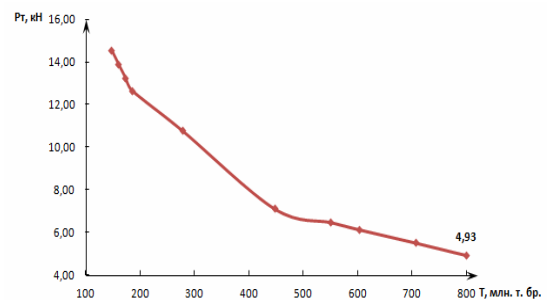
Рис. 12. Графік загального зменшення сили притиснення із врахуванням всіх факторів
