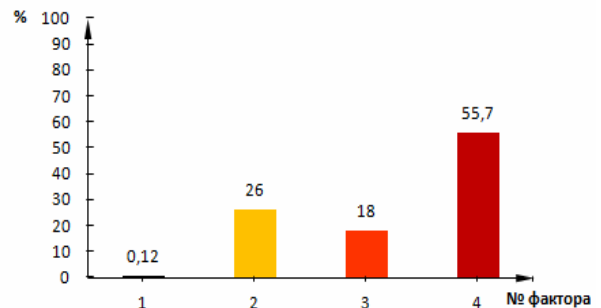
Рис. 11. Вплив факторів на силу притиснення рейки до підрейкової основи в рейковому скріпленні типу КПП-5:
