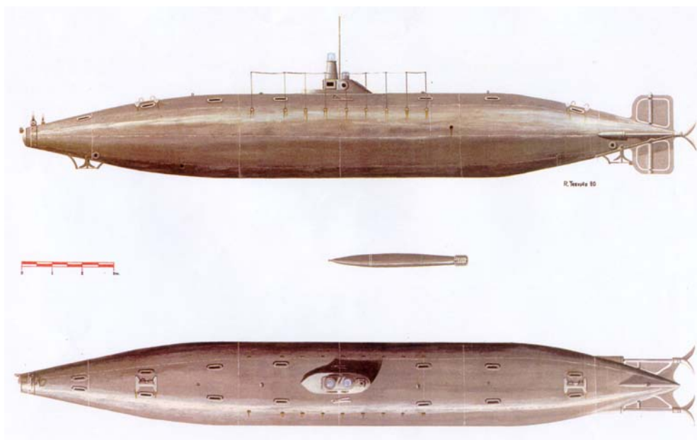
План-схема подводной лодки Пералья
