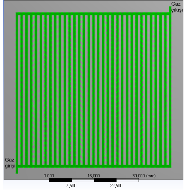
Şekil 1. Paralel akışlı akım toplayıcı plaka (Parallel-flow current collector plate)
