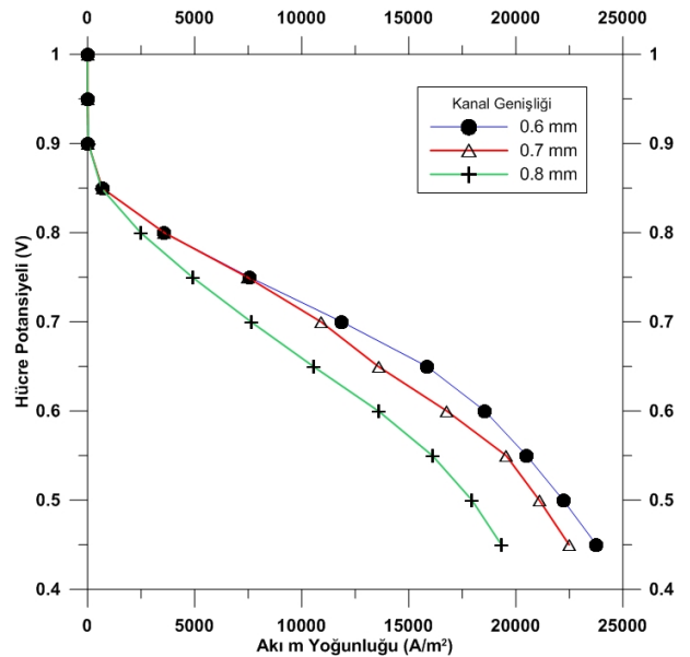
Şekil 7. T =353 K, P =2 atm çalışma şartları ve farklı kanal genişliklerinde V-I eğrisi(T =353 K, P =2 atm VI curve in working conditions and different channel width)
