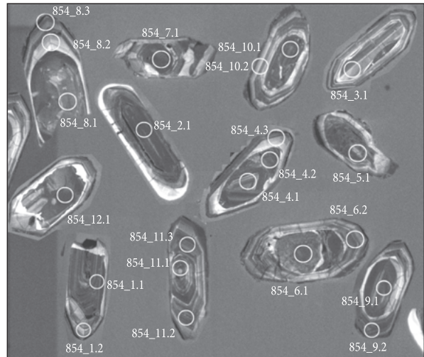
Рис. 3. Мікрофотографії полірованих зрізів кристалів циркону із тоналіту другої фази інтрузії Добропільського масиву. Катодолумінесцентні зображення
