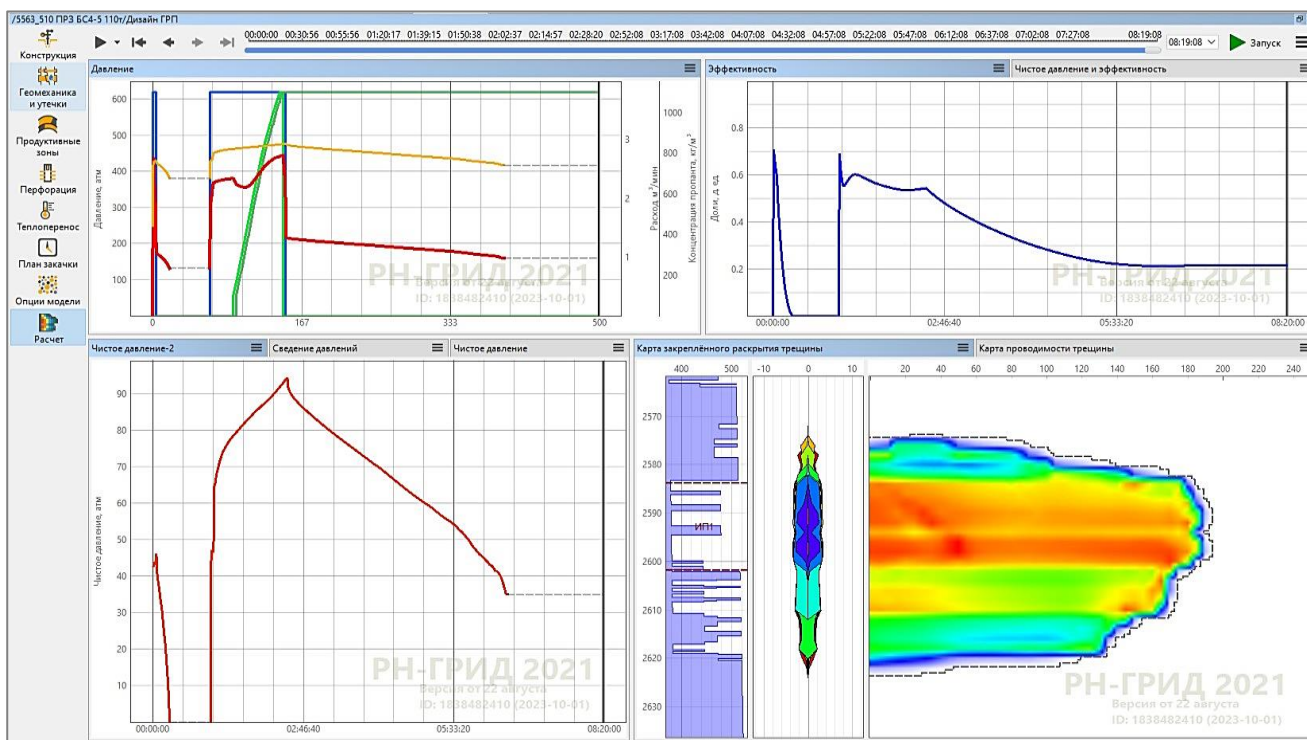
Рисунок 4. Изменение давления, эффективности, раскрытия трещины при закачке 300 м 3 жидкости
