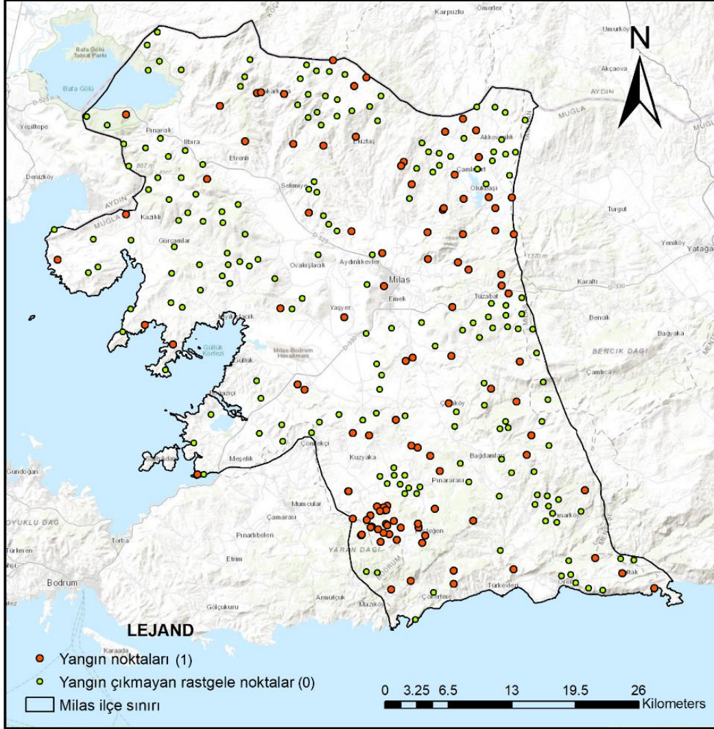
Şekil 3: Alandaki yangın varlık ve yokluk noktaları
