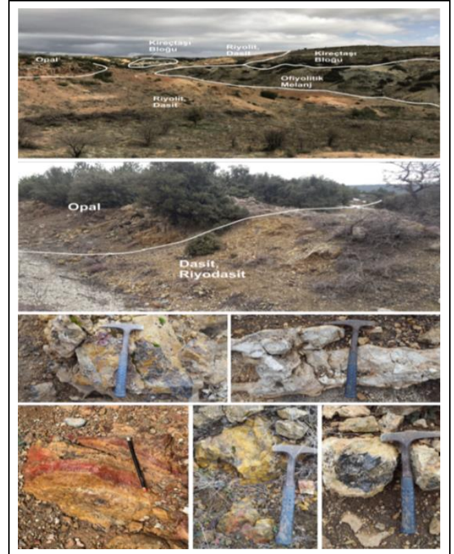
Şekil 3. Keçiborlu-Değirmendere Köyü ve çevresindeki farklı renklerdeki opal oluşumları ve ilişkili jeolojik birimler.
