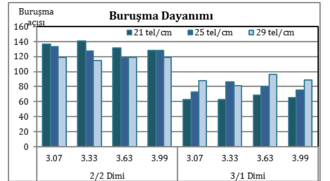
Şekil 5. Buruşma geri dönüşüm açısı testi sonuçları.
