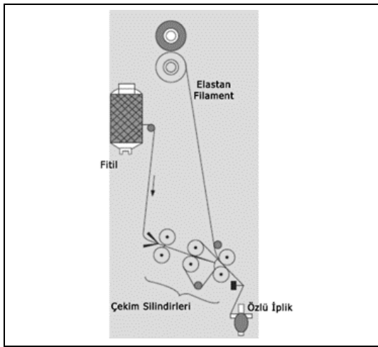
Şekil 1. Ring makinesinde elastan özlü iplik üretim prensibi [11].
