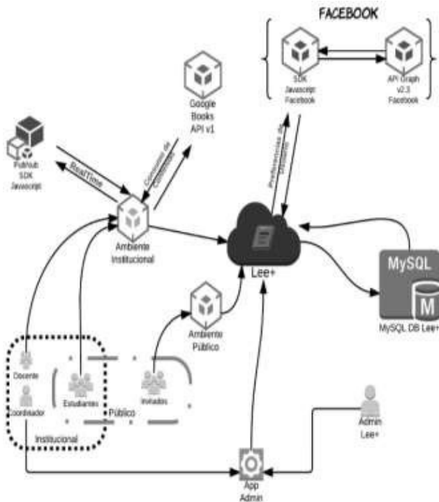
Figura 10. Arquitectura Lee+.
