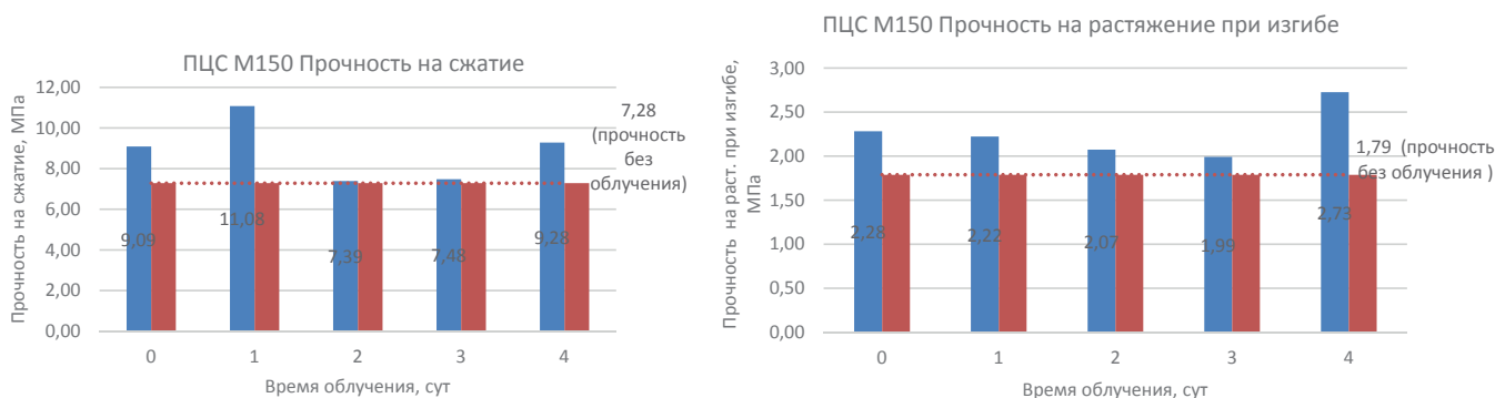
Рис. 1. Результаты определения прочности на сжатие и растяжение при изгибе образцов ПЦС М150
