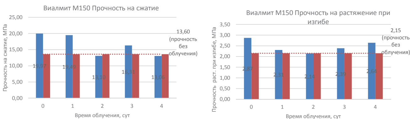
Рис. 2. Результаты определения прочности на сжатие и растяжение при изгибе образцов Виалмит М150
