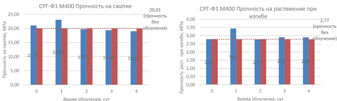
Рис. 4. Результаты определения прочности на сжатие и растяжение при изгибе образцов SRG-F1 M400
