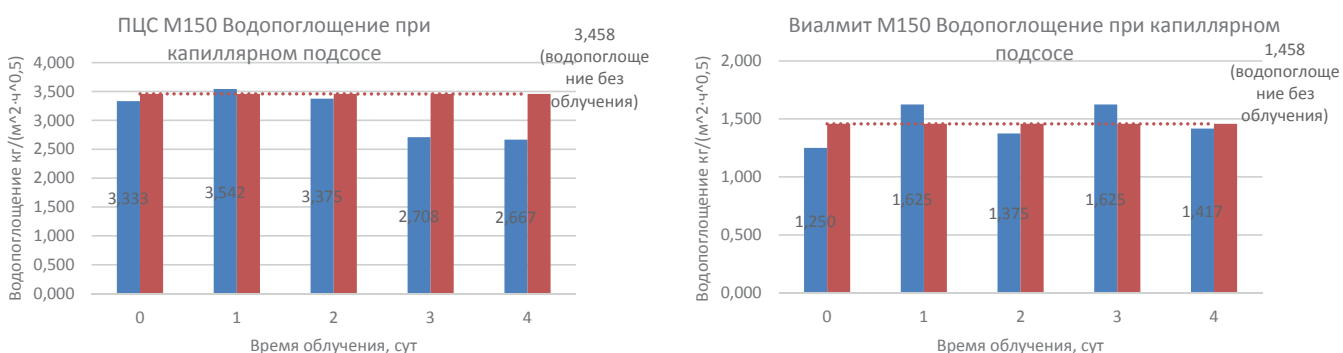
Рис. 5. Результаты определения водопоглощения при капиллярном подсосе образцов ПЦС М150 и Виалмит М150
