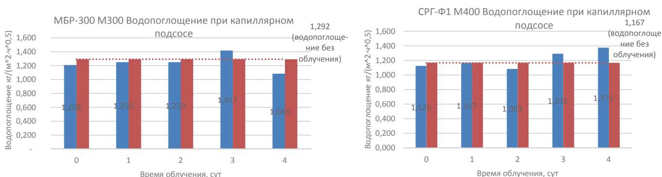
Рис. 6. Результаты определения водопоглощения при капиллярном подсосе образцов МБР-300 М300 и SRG-F1 M400
