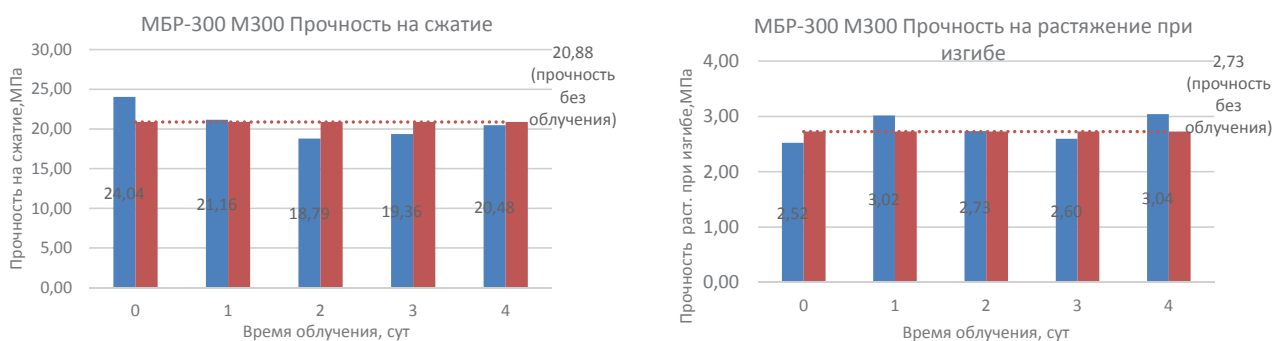
Рис. 3. Результаты определения прочности на сжатие и растяжение при изгибе образцов МБР-300 М300
