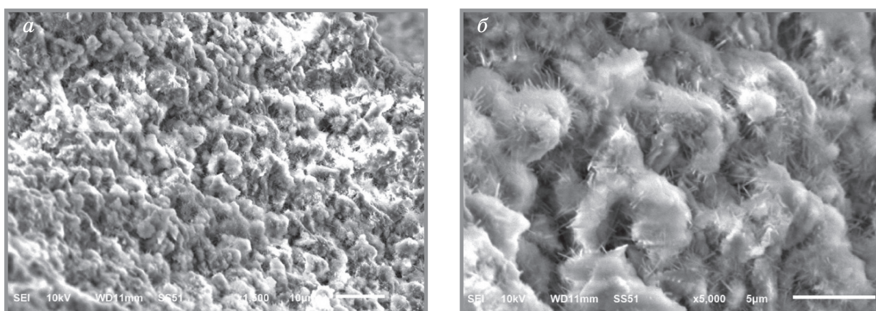
Рис. 7. Электронно-микроскопические снимки структуры образцов ЦПР без воздействия: а) увеличение \times 5000 , масштаб отрезка 5 мкм, б) увеличение \times 1500 , масштаб отрезка 10 мкм
