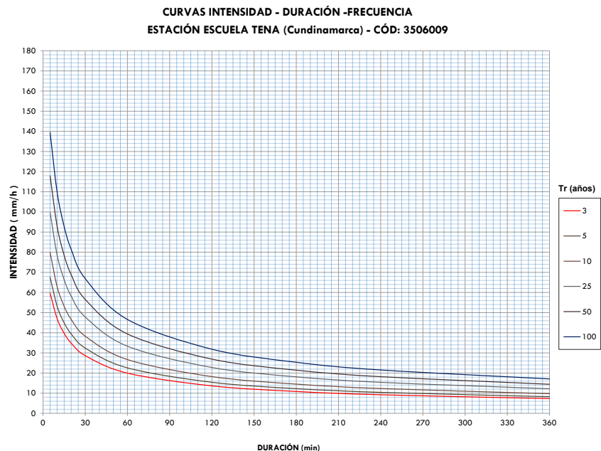
Figura 2. Ejemplo de curva IDF
