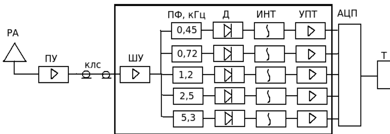
Рис. 1. Структурная схема ОНЧ-пеленгатора
