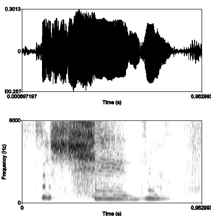
FIGURA 1 – Espectrograma da palavra vestido , pronunciada como θισυσιδY, pelo informante T, de 1:6:18.
