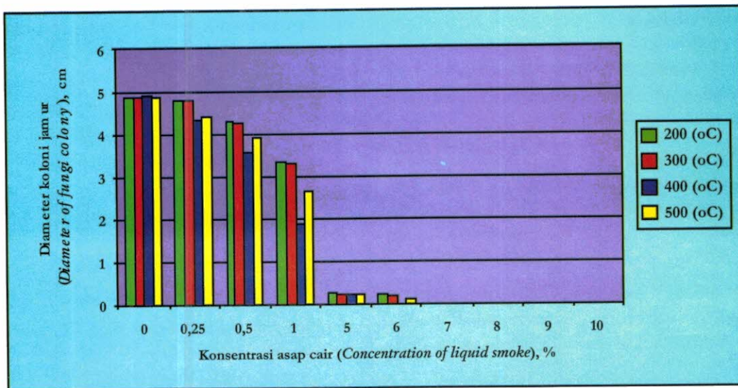
Gambar 2. Ilustasi histogram rata-rata diameter koloni cendawan Colletotrichum gloeosporoides pada hari ke tujuh di kultivasi pada media PDA dengan perlakuan asap cair pada berbagai suhu destilasi kering ( B, ^\circ C )
