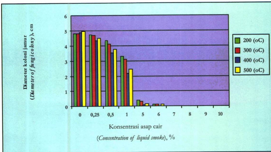
Gambar 3. Ilustasi histogram rata-rata diameter koloni cendawan Colletotrichum gloeosporoides pada hari ke tujuh di kultivasi pada media PDA dengan perlakuan asap cair pada berbagai suhu destilasi kering ( B, ^\circ C )
