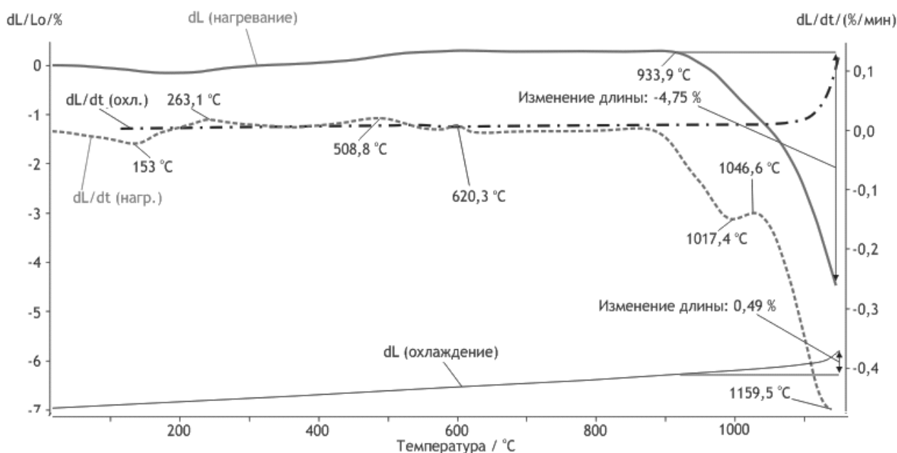
Рис. 3. Дилатогрaмма массы оптимального состава
